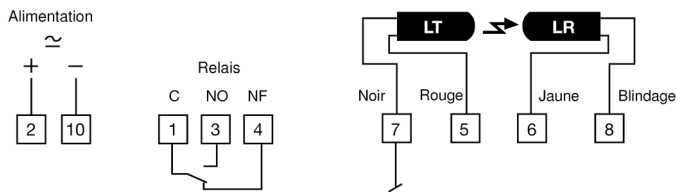
Sortie relais – PA 10 A/B 51X
